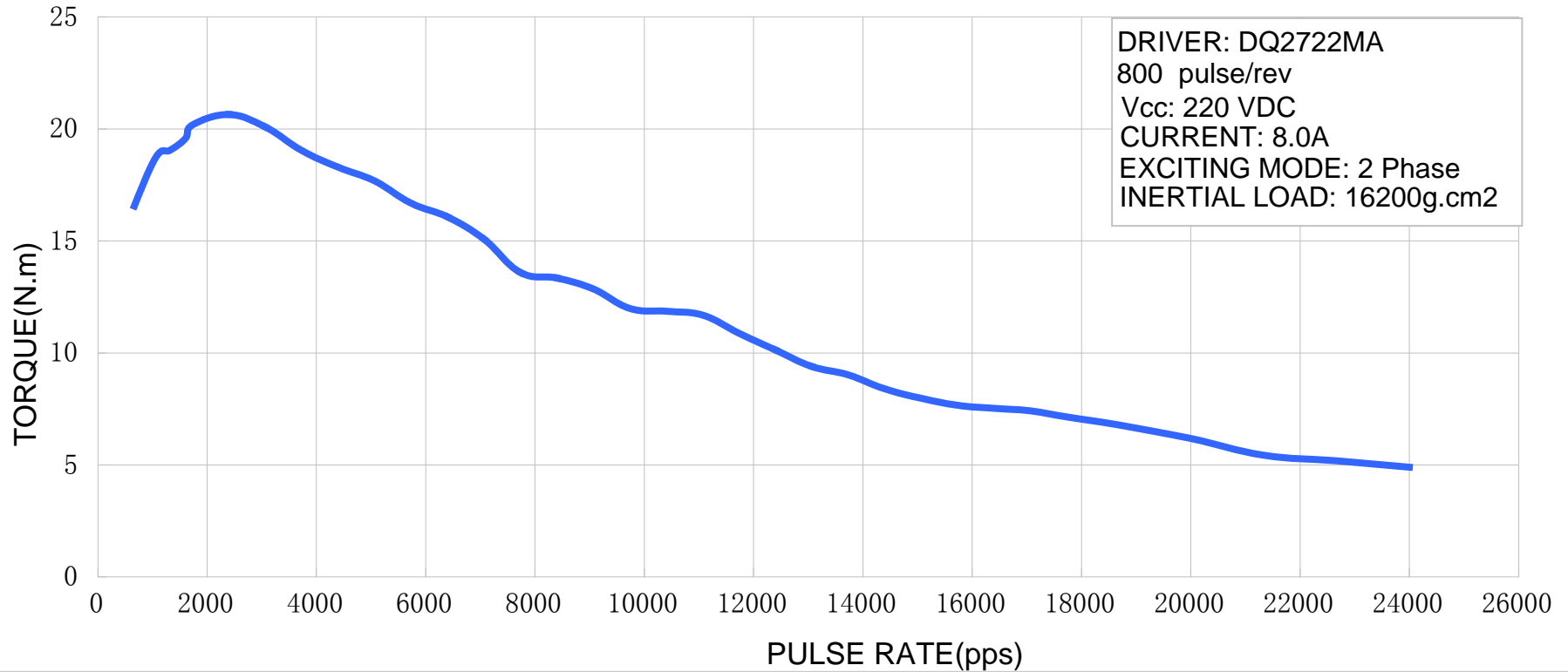
110BYGH201-001 Torque Curve
